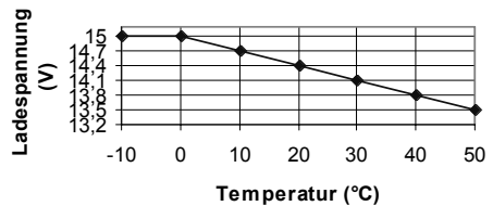
Temperaturabhängigkeit der Gasungsspannung einer 12V-Blei-Gel-Batterie
