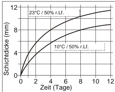
Diagramm 1: Durchhärtageschwindigkeit für Sikaflex®-291
